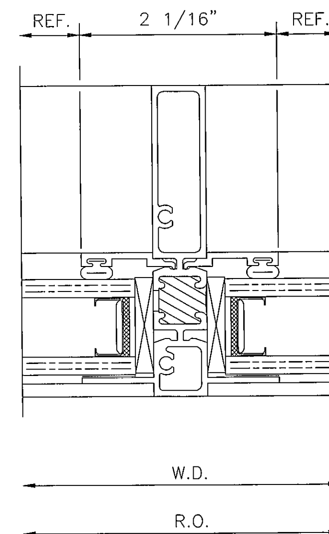
48 MUNTIN
