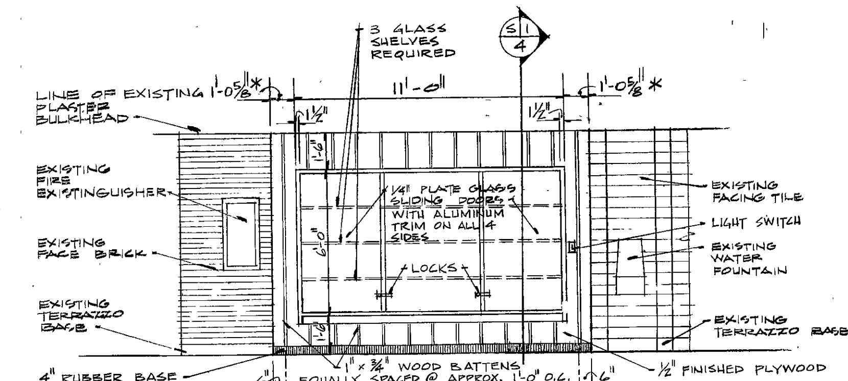
ELEVATION
