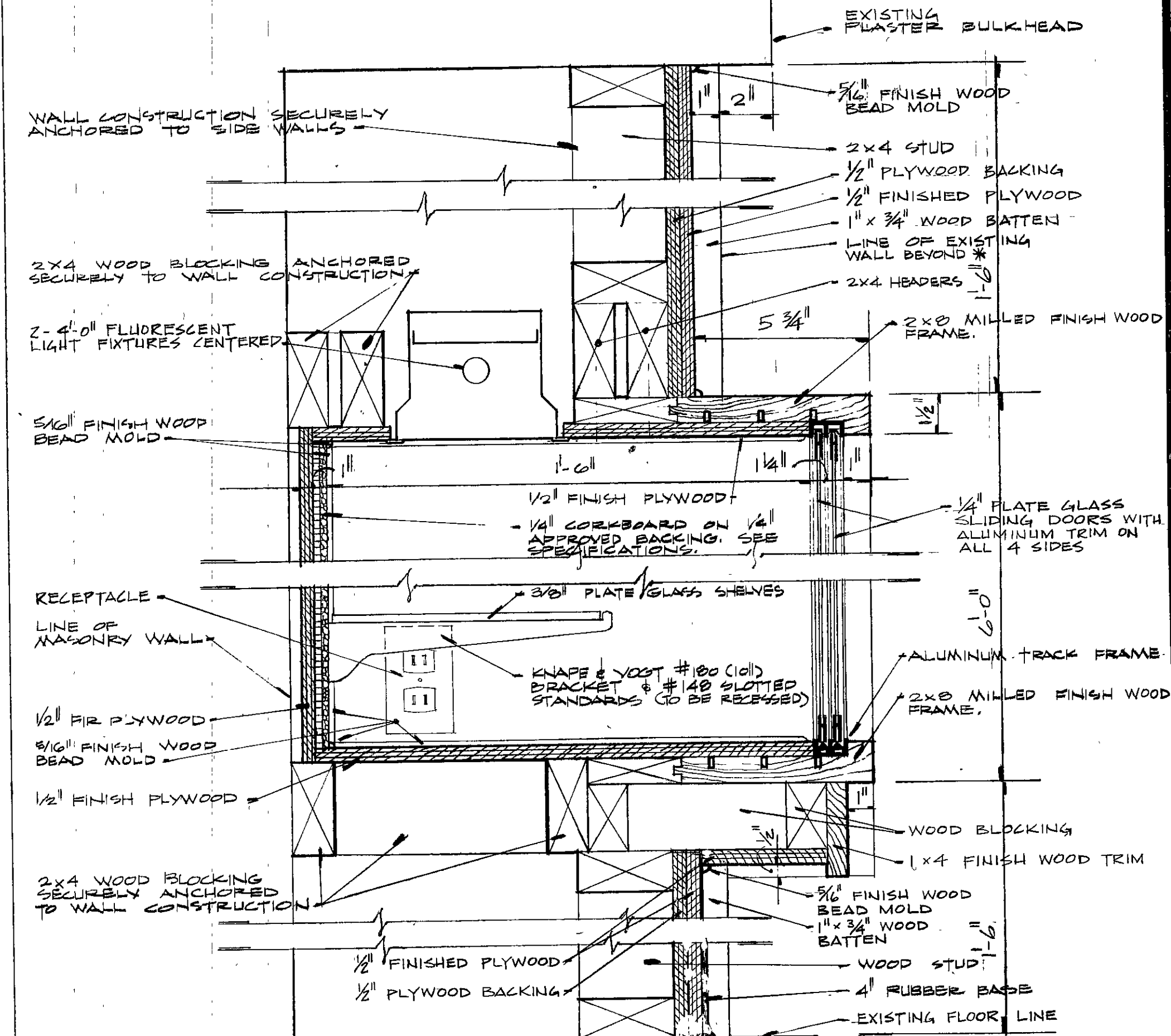
SECTION 51 SCALE: 2" = 1'-0" 4
