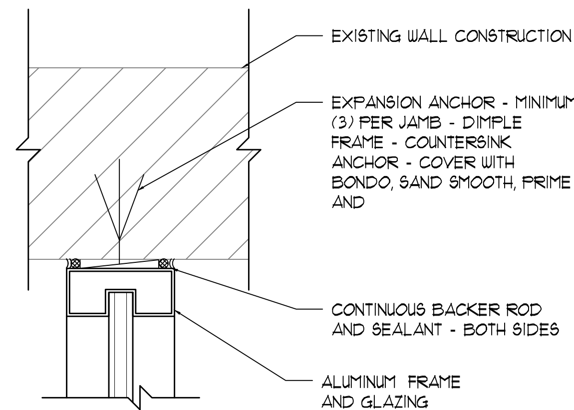
5 JAMB DETAIL 3" x 1'-0"
